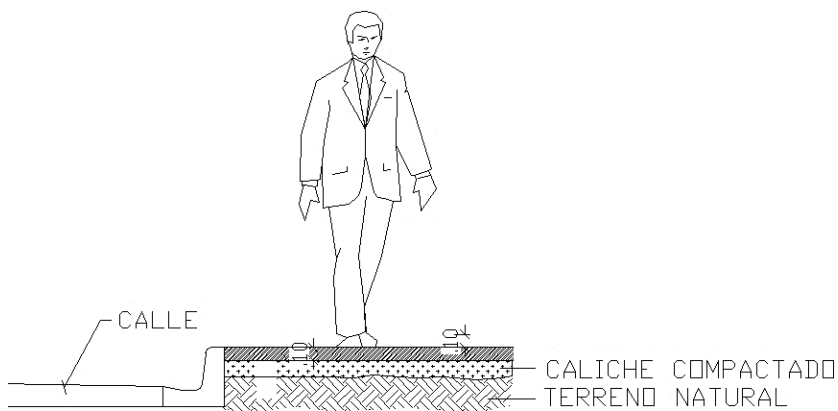
01 DETALLE DE ACERAS
